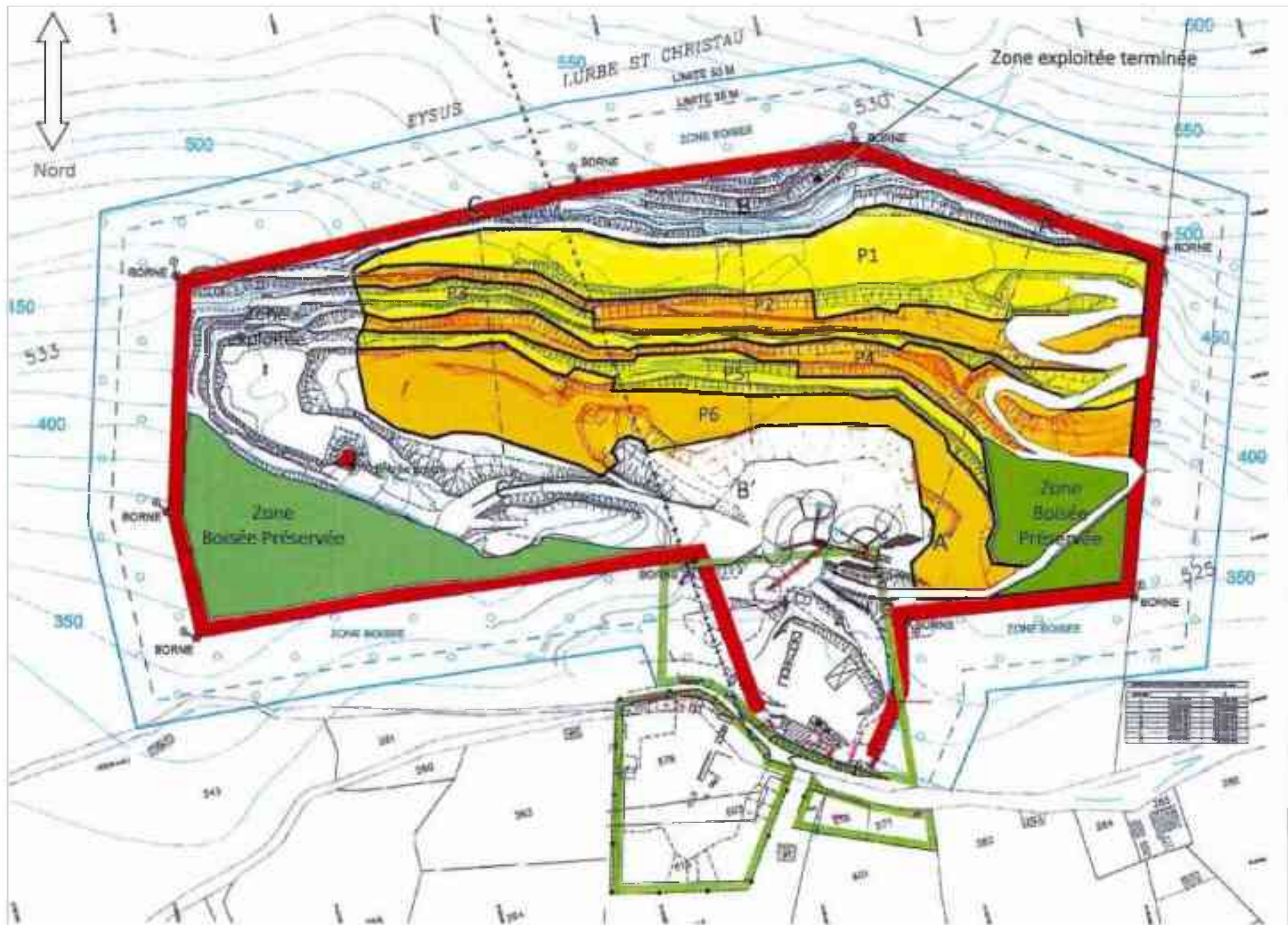
PL.3 : Plan d'exploitation de la carrière de Lurbe-Saint-Christau - Echelle approximative : 1 / 3300
