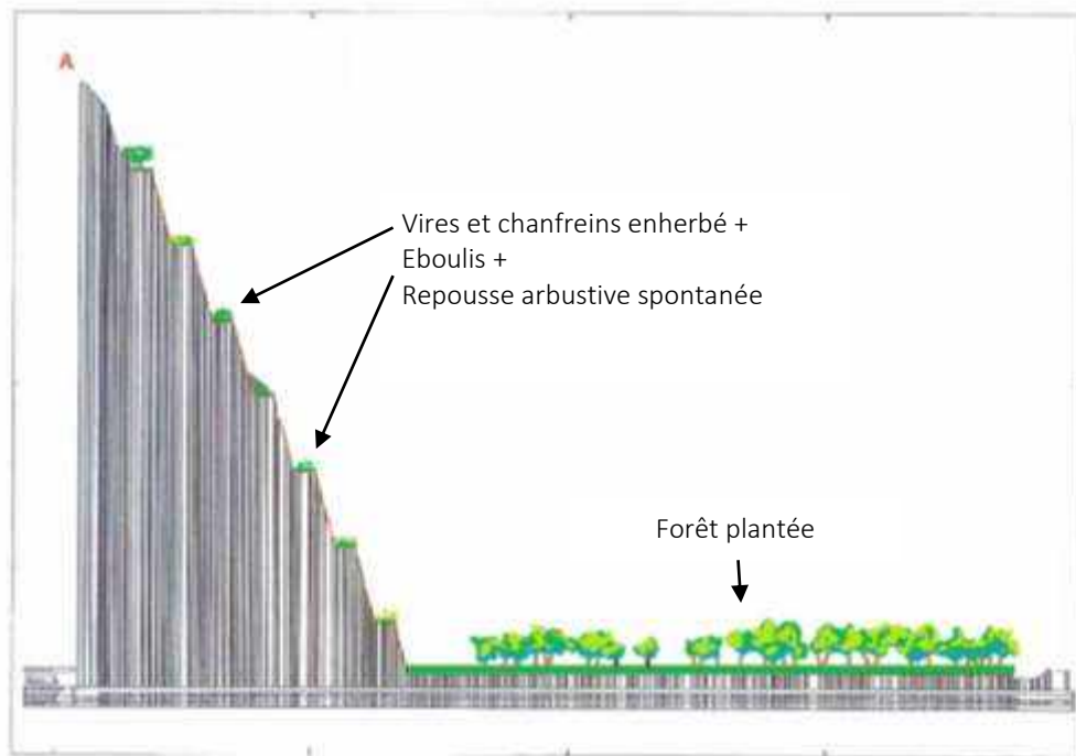
PL.18 : Coupes de la remise en état de la carrière de Lurbe-Saint-Christau
