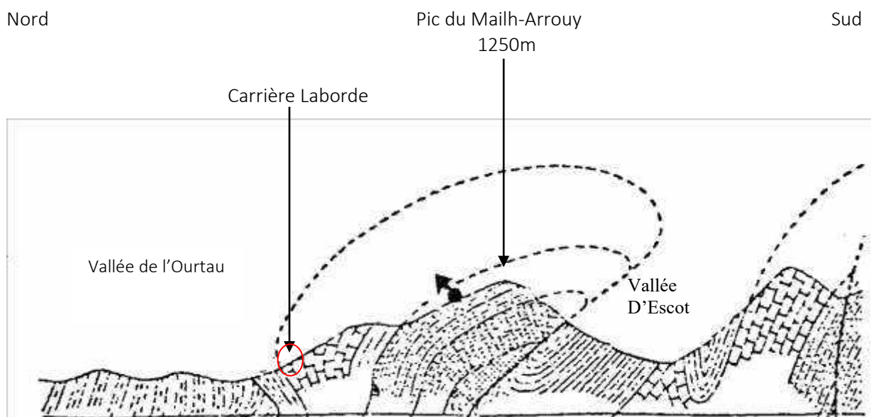
PL.9 : Coupe géologique à travers le chaînon du Mailh-Arrouy de P. Viennot
