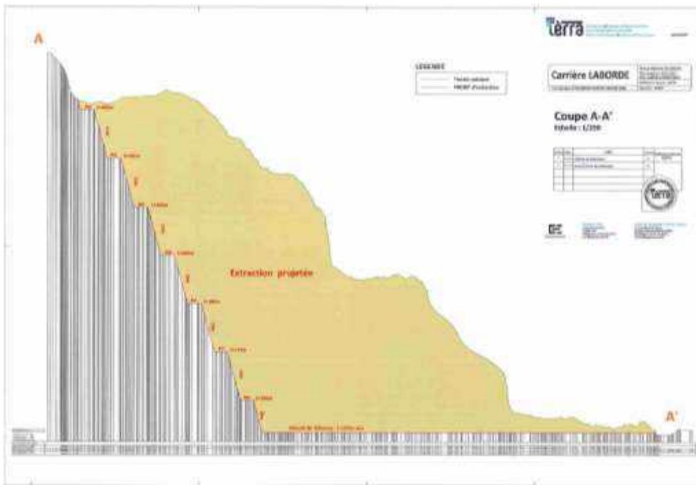
PL.5 : Profils topographiques des matériaux restant à extraire
