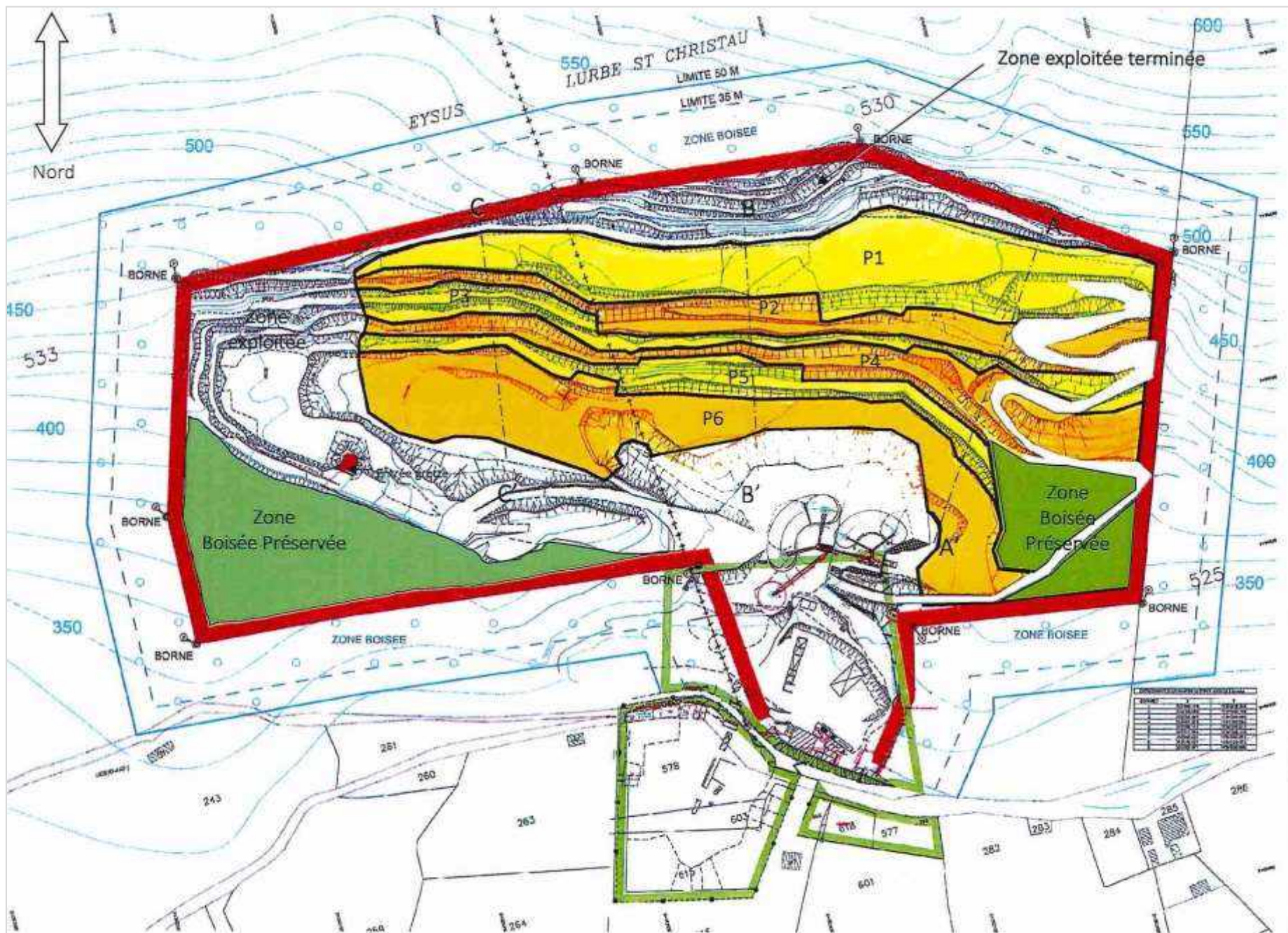
PL.6 : Plan d'exploitation de la carrière de Lurbe-Saint-Christau - Echelle approximative : 1 / 3300
