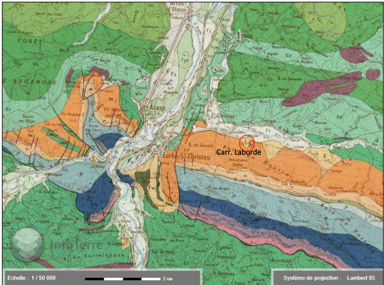
PL.8 : Extrait de la carte géologique d'Orlon-Sainte-Marie au 1 / 50 000 (B.R.G.M.)
