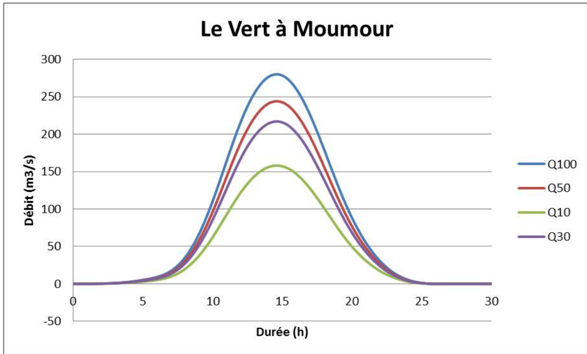
Fig. 44. Hydrogrammes du Vert à Moumour
