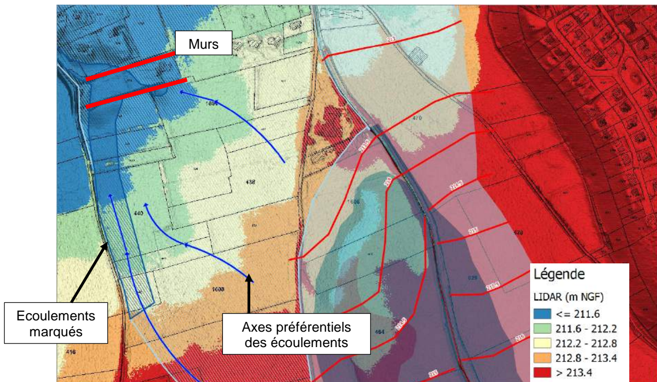
Fig. 55. Ruissellement superposé au LIDAR sur le plateau
