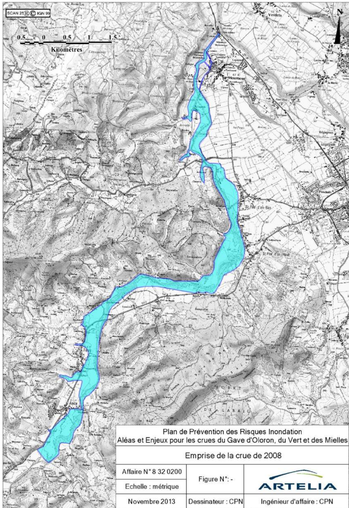
Fig. 31. Emprise de la crue de 2008 sur le bassin versant du Vert
