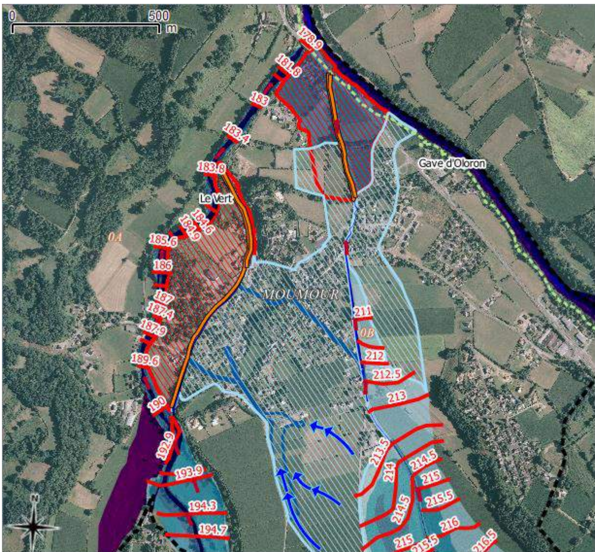
Fig. 72. Zone aval endiguée : Ruissellement (hachures bleues) et rupture de digue (hachures rouges)
