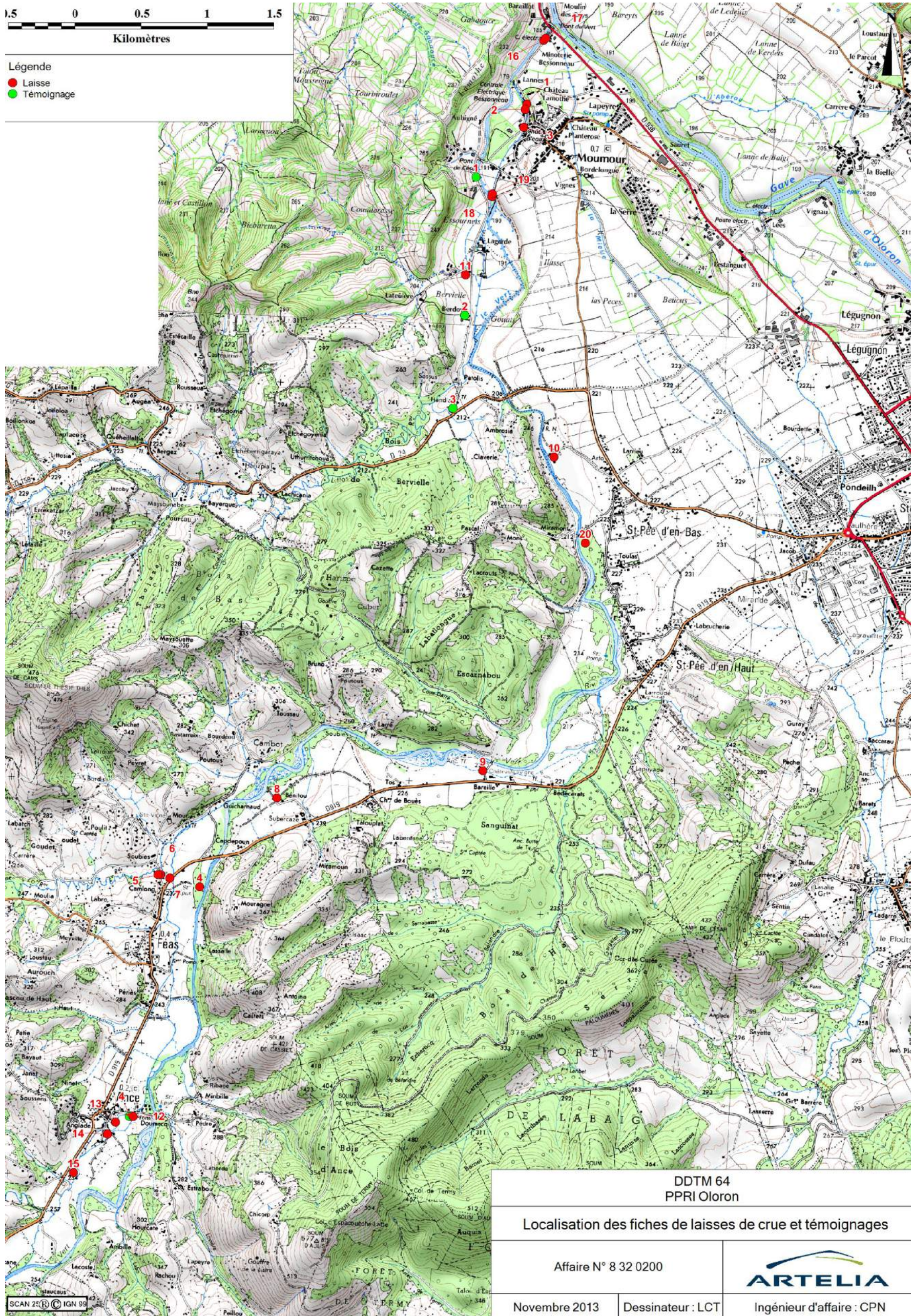
Fig. 8. Localisation des fiches de laisses de crue et de témoignage
