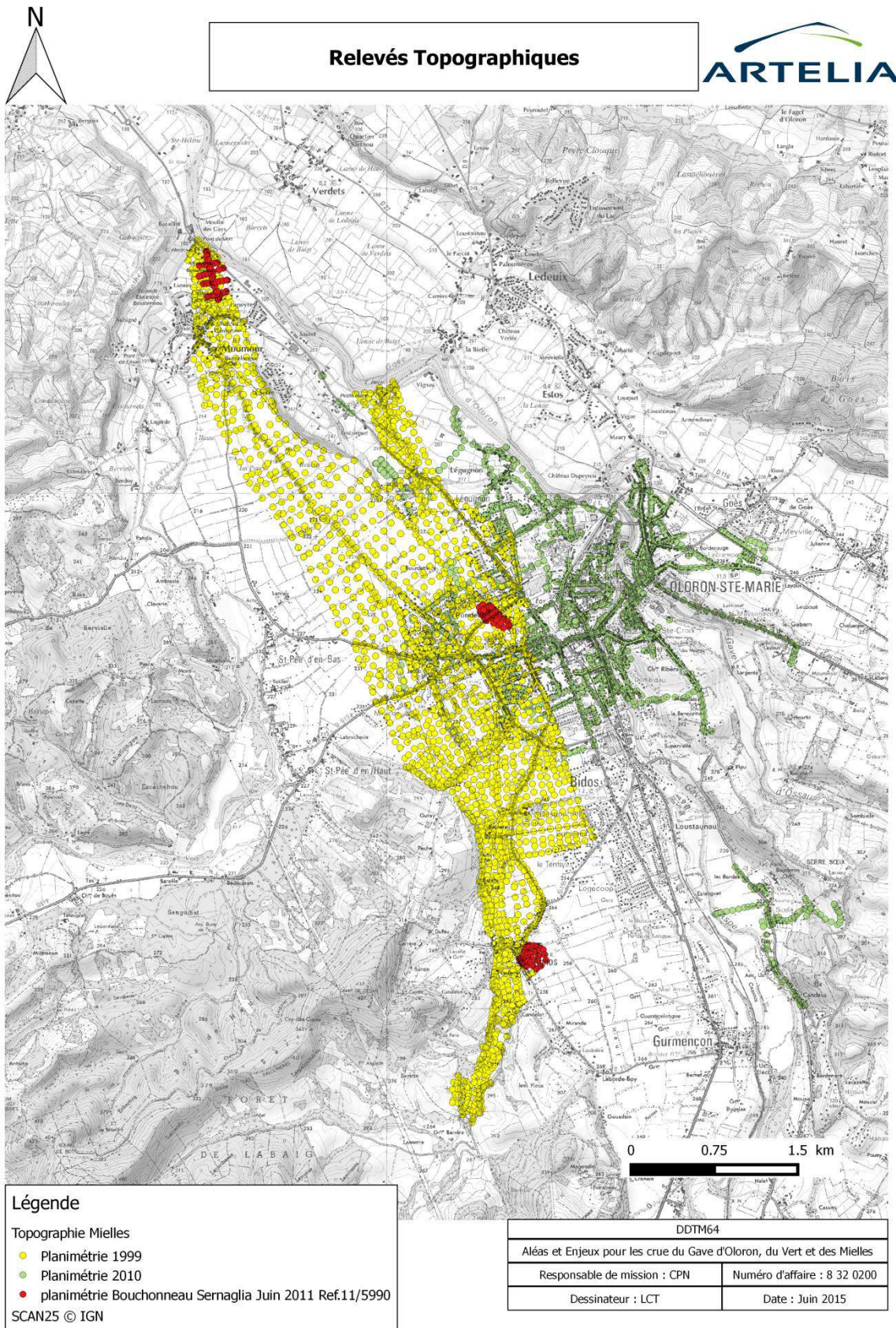
Fig. 2. Topographie des Mielles
