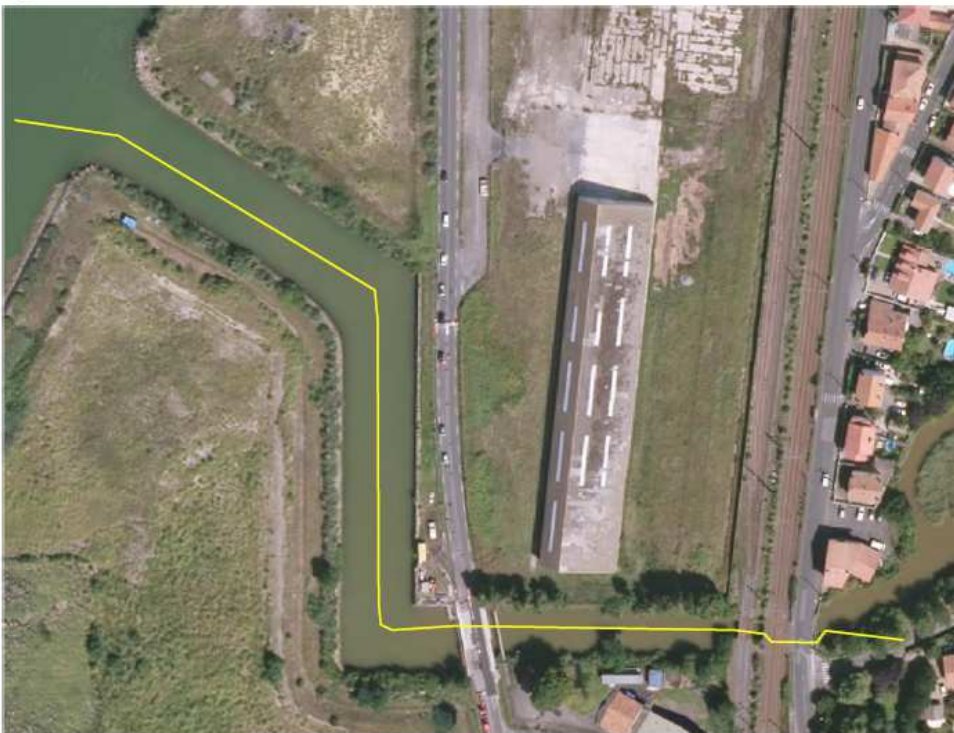
Figure 6 : Tracé de la nouvelle canalisation dans le lit du ruisseau du Moulin d'Esbouc
