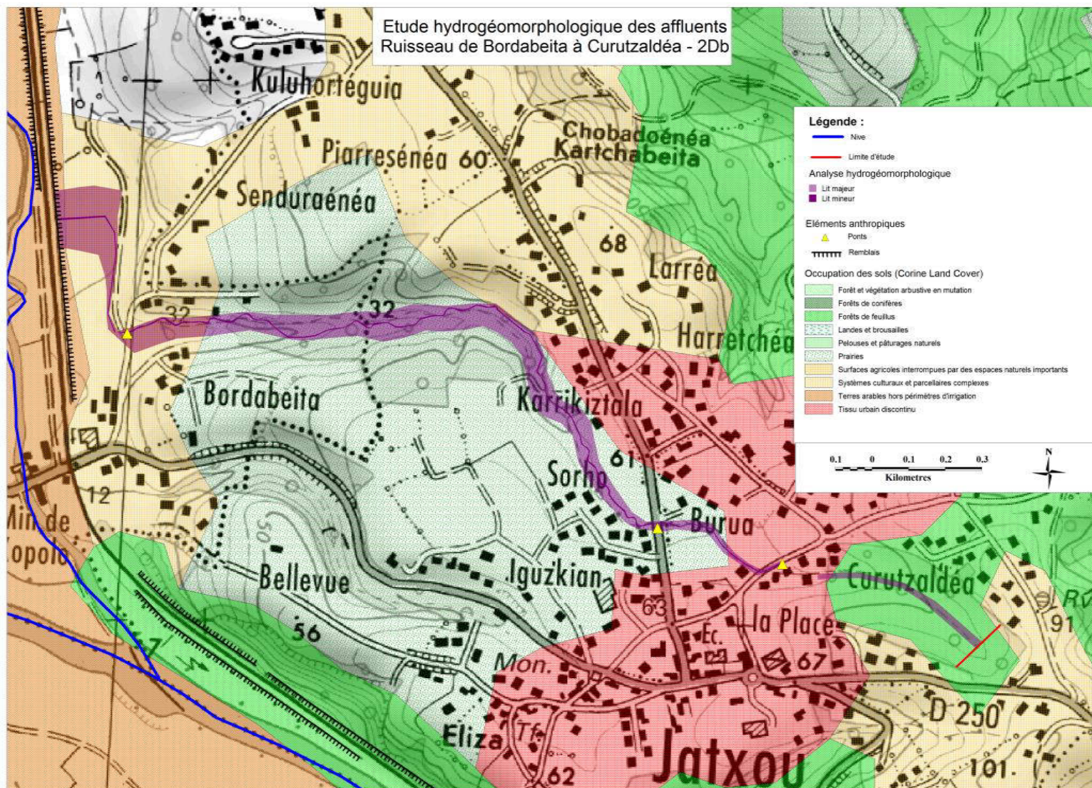
Figure 7 : Tracé du lit majeur du ruisseau de Bordabeita à Curutzaldea selon la méthode hydrogéomorphologique
