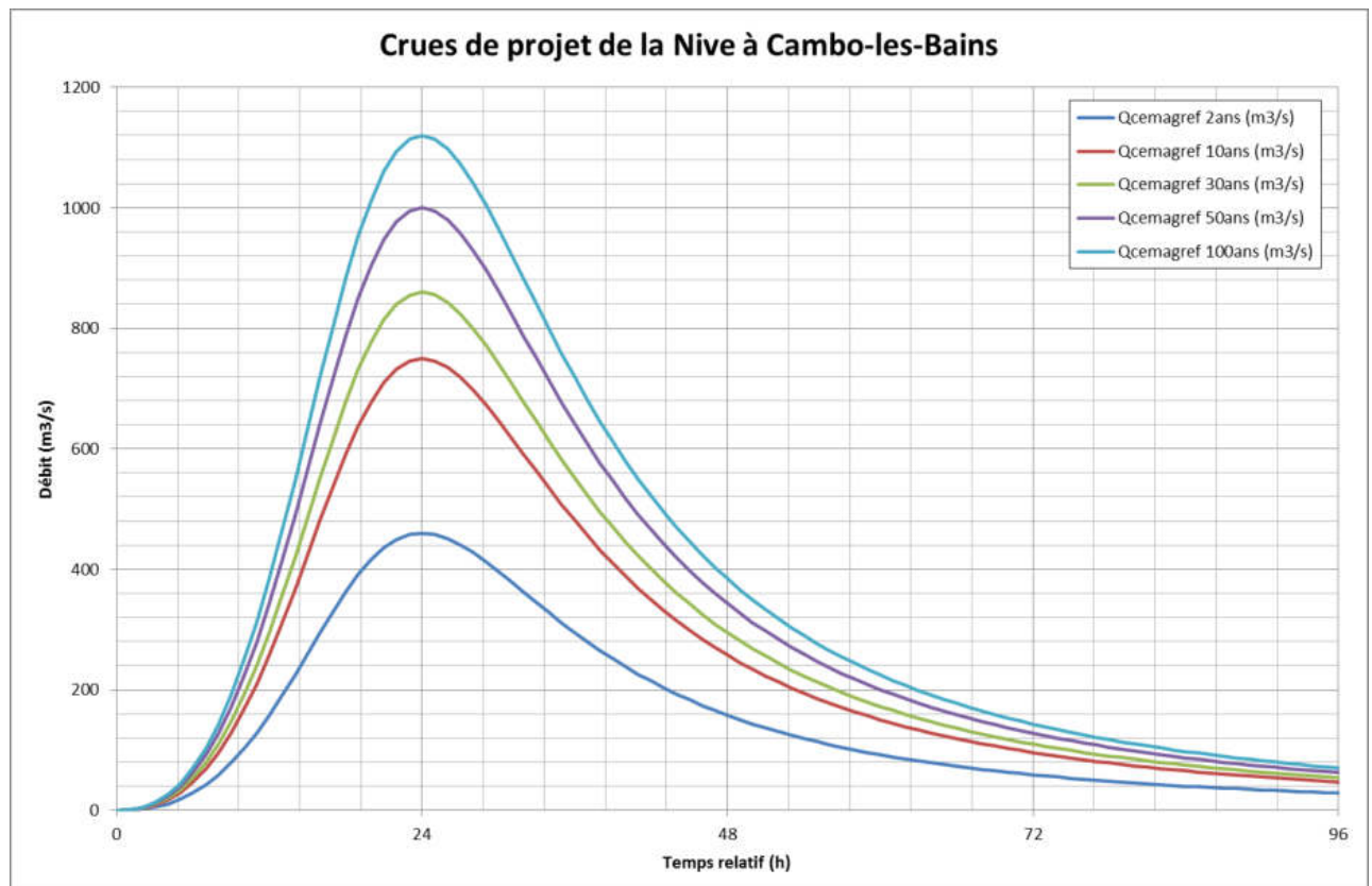
Figure 6 : Hydrogrammes des crues de projet de la Nive à Cambo-les-bains
