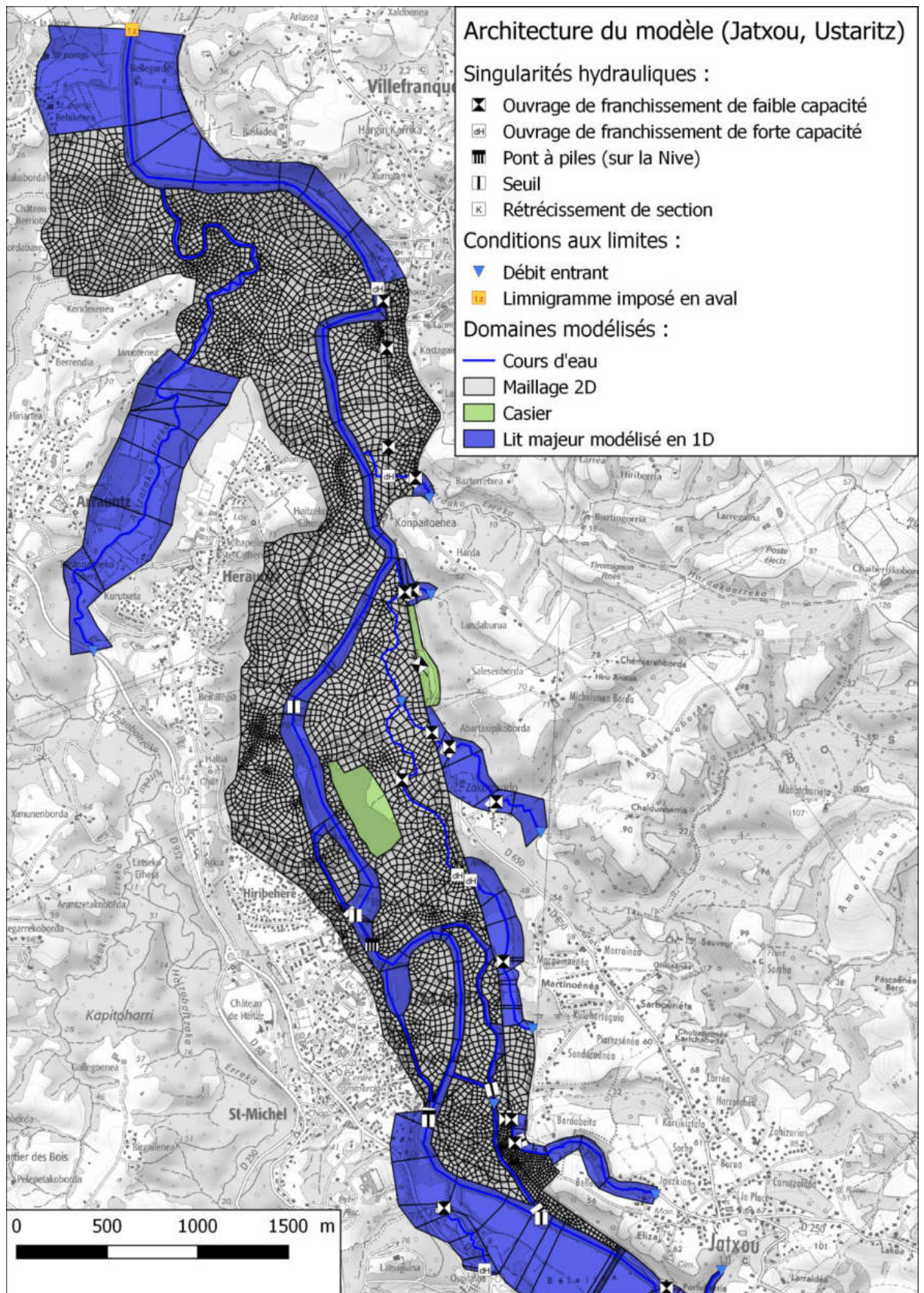
Figure 9 : Architecture du modèle au droit de Ustaritz
