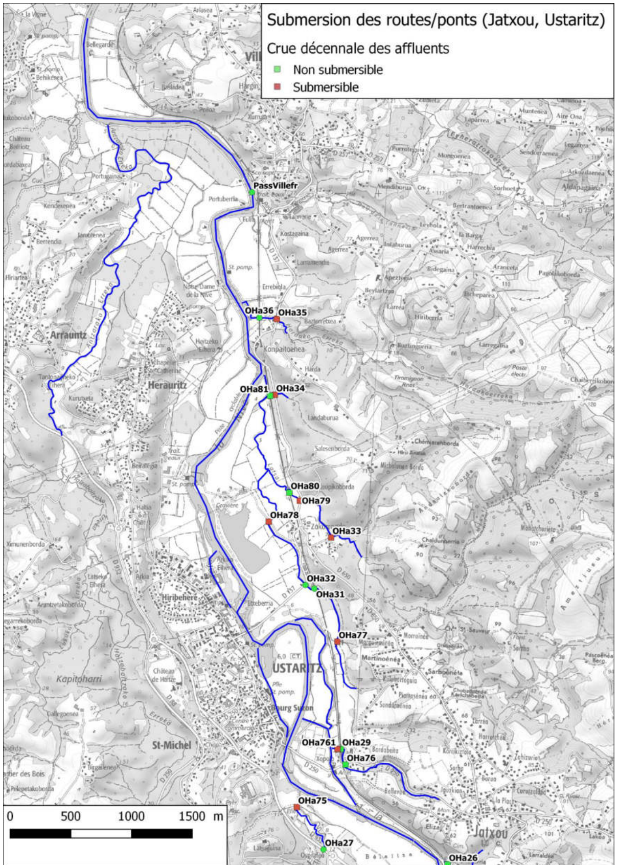
Figure 13 : Submersion des routes/pont au cours de la crue centennale des affluents – Ustaritz
