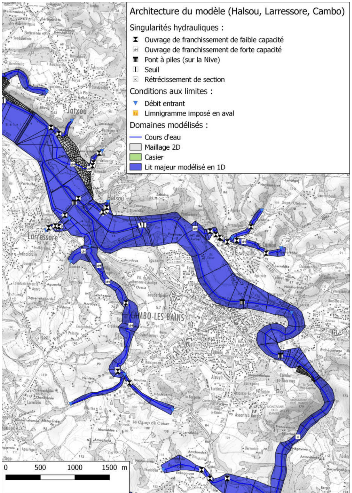
Figure 9 : Architecture du modèle au droit de Larressore
