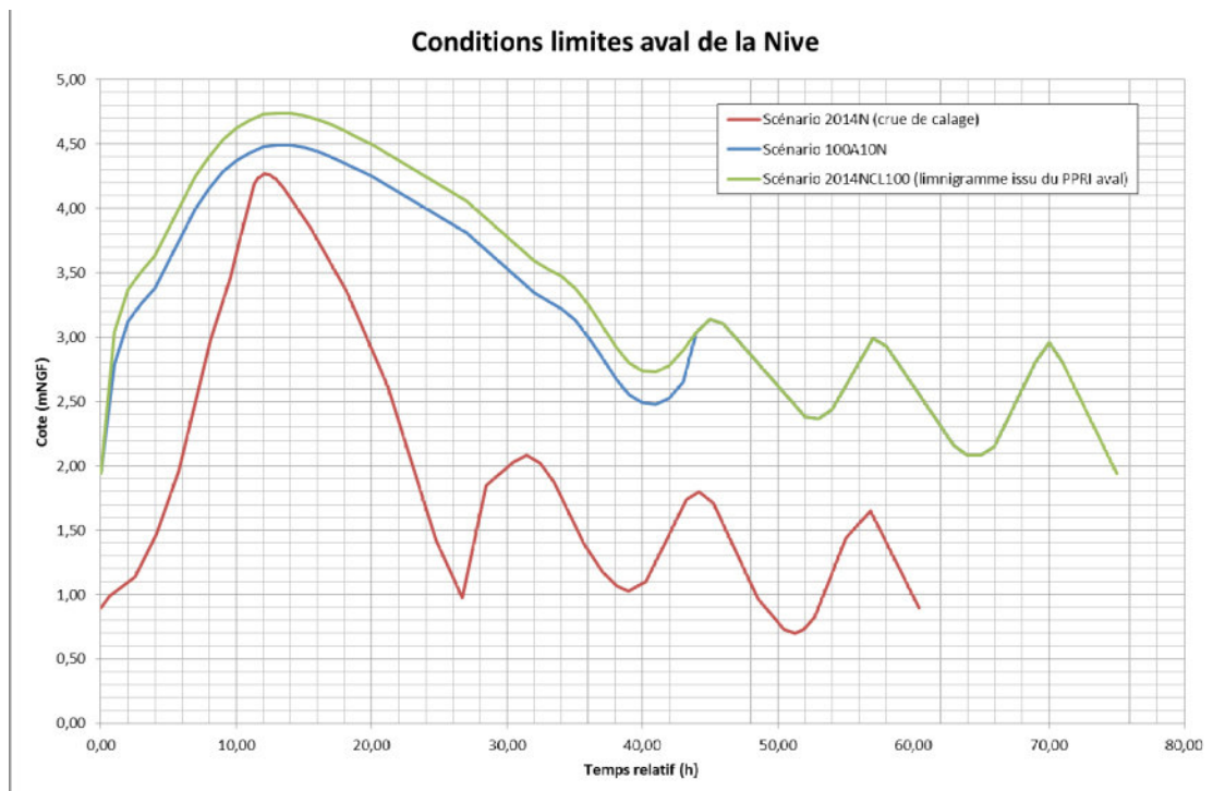
Figure 11 : Conditions à la limite aval de la Nive
